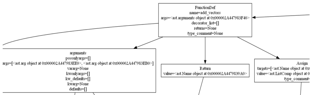
Рисунок 5 – Фрагмент визуализированного AST
