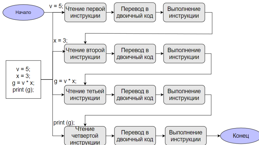
Рисунок 2 – Реализация интерпретатора
